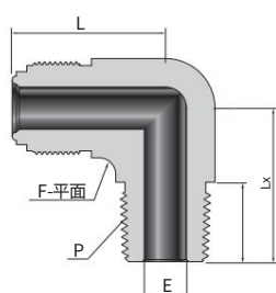
GFS 轉NPT 陽螺紋彎頭
