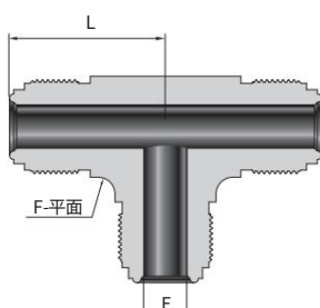
GFS 三通
